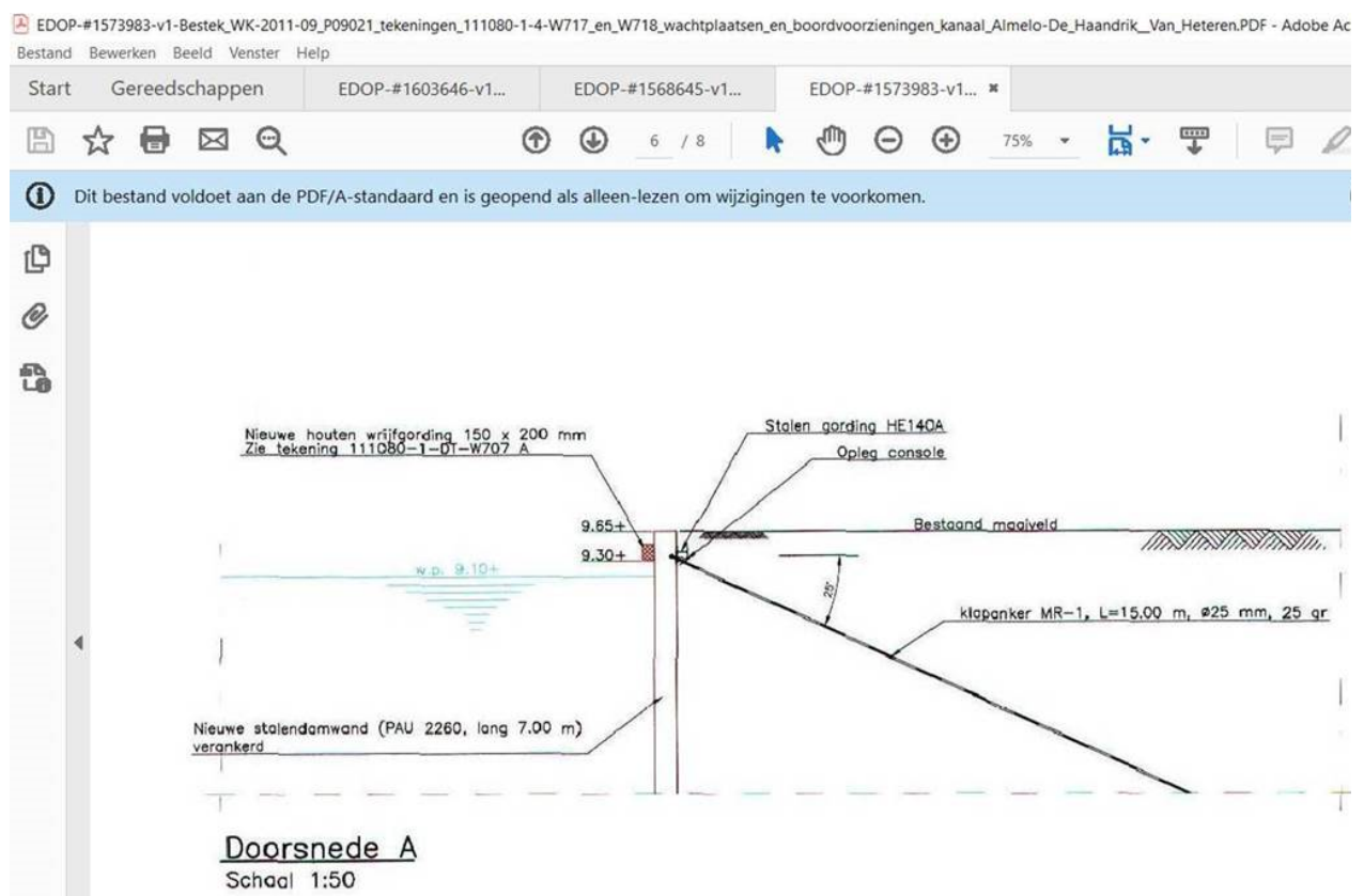
Figuur 1 Technische tekening klapanker Bron:provincie Overijssel
